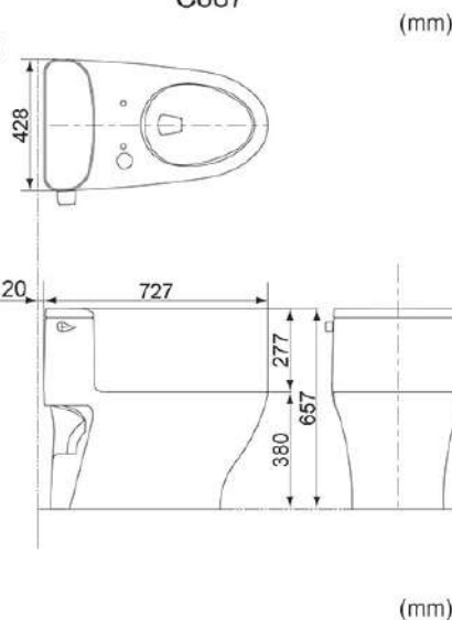
Sơ đồ lắp đặt sản phẩm C887***
