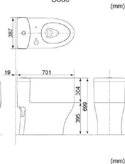
Sơ đồ lắp đặt sản phẩm C889***
